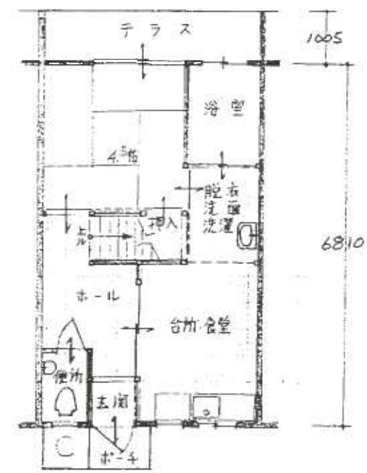
1階平面図
