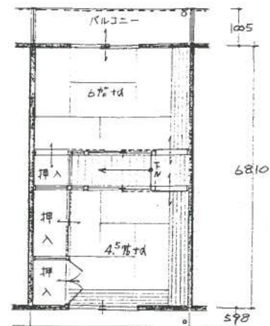
2階平面図
