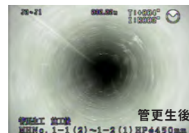
工事例2)老朽化した下水道管を内側から補強する管更生工事
