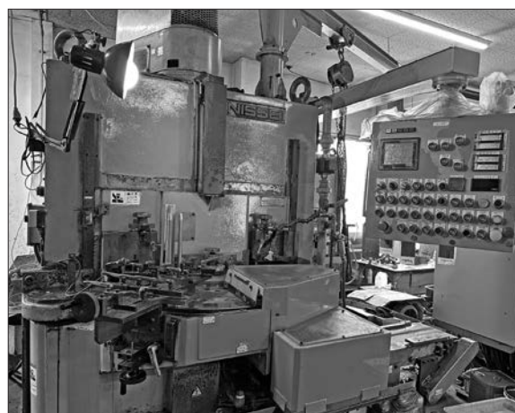
● 立型両頭平面研削盤 V-5P
