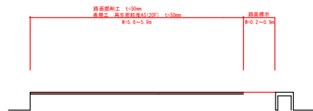
標準断面図 1:30
