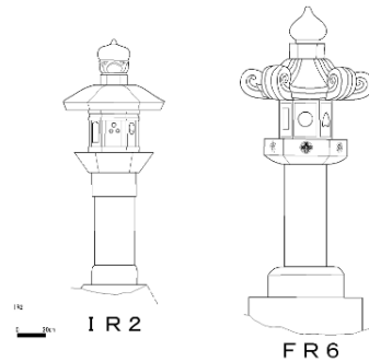
図 12 石灯籠測量図 I R 2・F R 6
