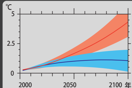
2081年~2100年の平均気温 ■ 現状を上回る対策をしなかった場合 ▶▶ 2.6~4.8°C上昇 ■ 厳しい対策をした場合 ▶▶ 0.3~1.7°C上昇
