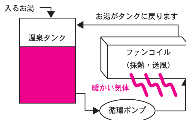
【図】温泉暖房システムの仕組み
